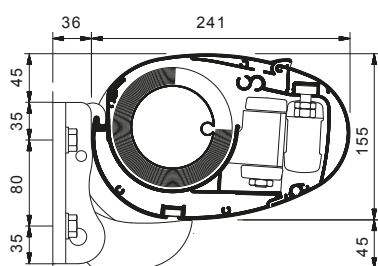
K350 Abmessungen
