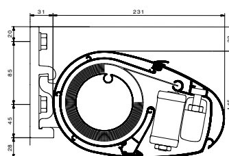
K200 Abmessungen
