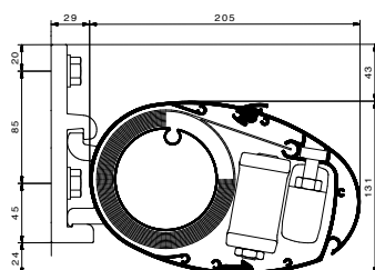
K100 Abmessungen
