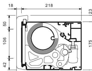
K450 Abmessungen
